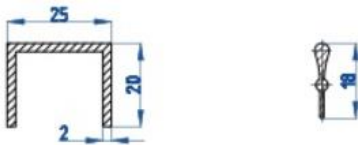
Сечение профиля рамки и перемычки Сечение профиля жалюзи
