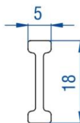
Сечение профиля жалюзи
