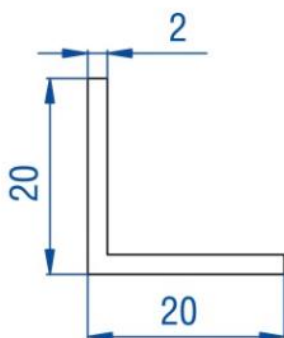
Сечение профиля рамки
