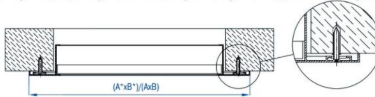
Монтаж решетки СЕЗОН ВР-ПП с помощью винтового соединения (отверстие Ø 3,5 мм), монтажные отверстия сверлятся по дополнительному заказу
