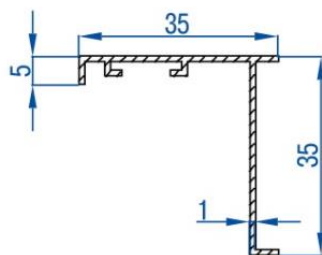
Сечение профиля рамки СЕЗОН ВР-Р, ВР-ПП
