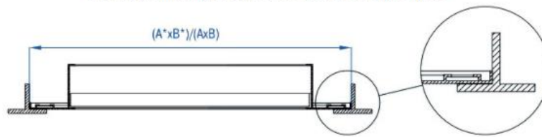
Расположение решетки СЕЗОН ВР-ПП на направляющих подвесного потолка «Армстронг»
