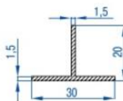
Профиль рамки СЕЗОН ВР-ПЯ
