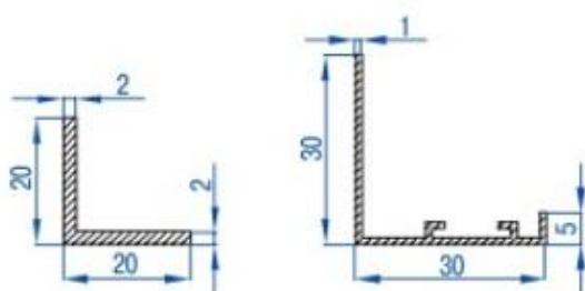
Профили рамки СЕЗОН ВР-Я
